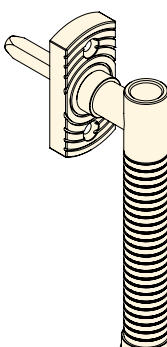
GROOVE 0404 G07 - 16Ø 0405 G07 - 19Ø
